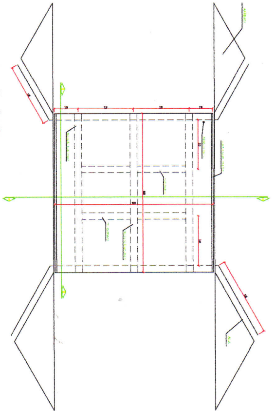
PLANTA BAIXA ESC. 1/100
