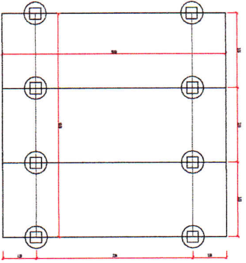
LOCAÇÃO DOS PILARES E TUBULÕES ESC. 1/100
