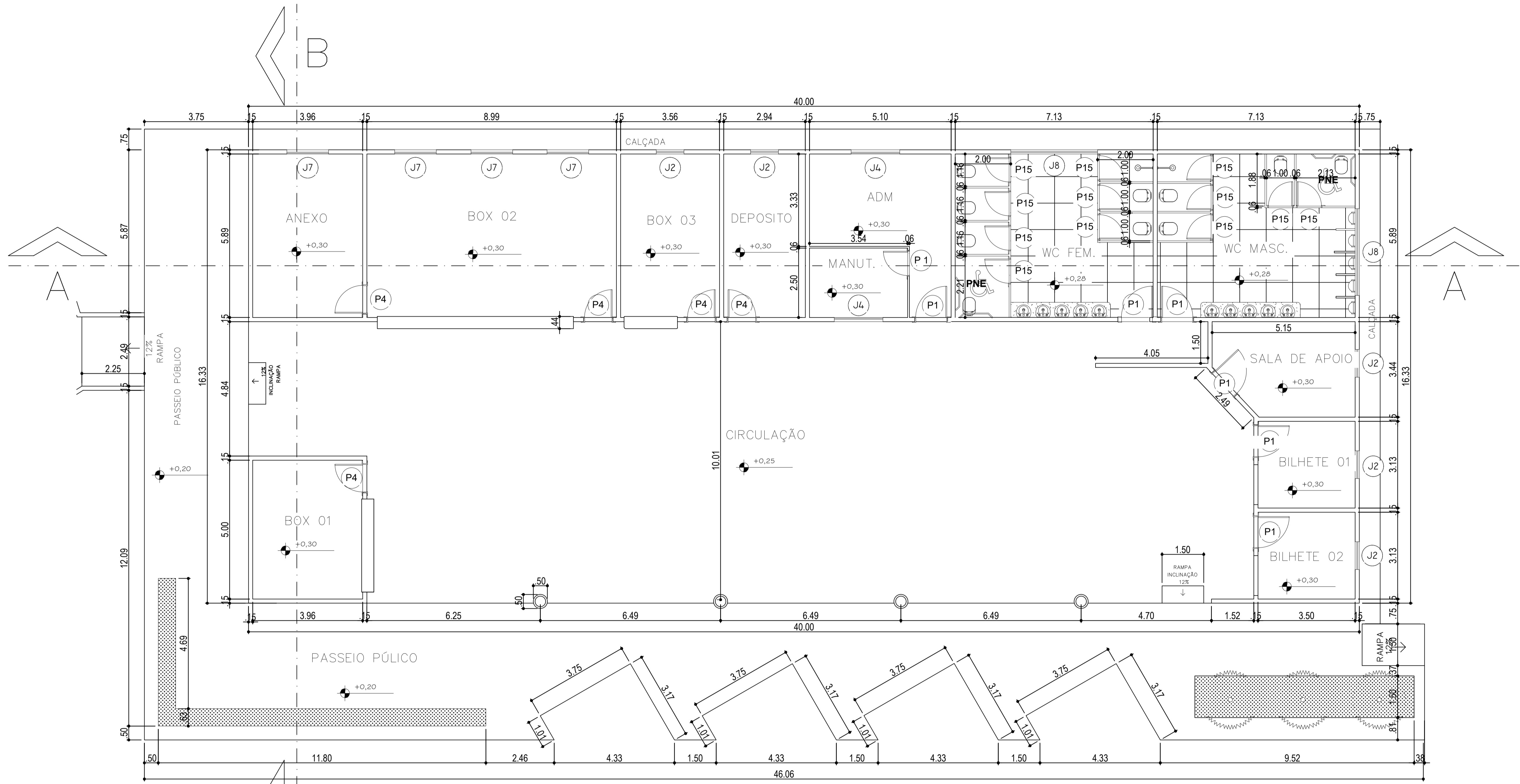
PLANTA BAIXA ESC.1/100
