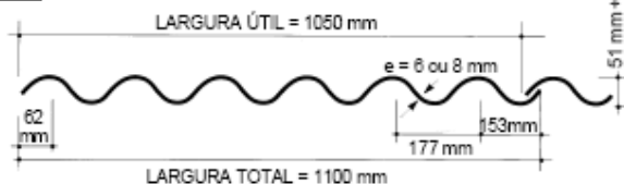
Figura Telhas onduladas de 6 mm e 8 mm - Seção transversal.
