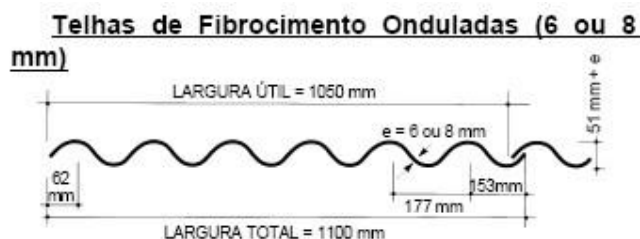
Figura Telhas onduladas de 6 mm e 8 mm - Seção transversal.
